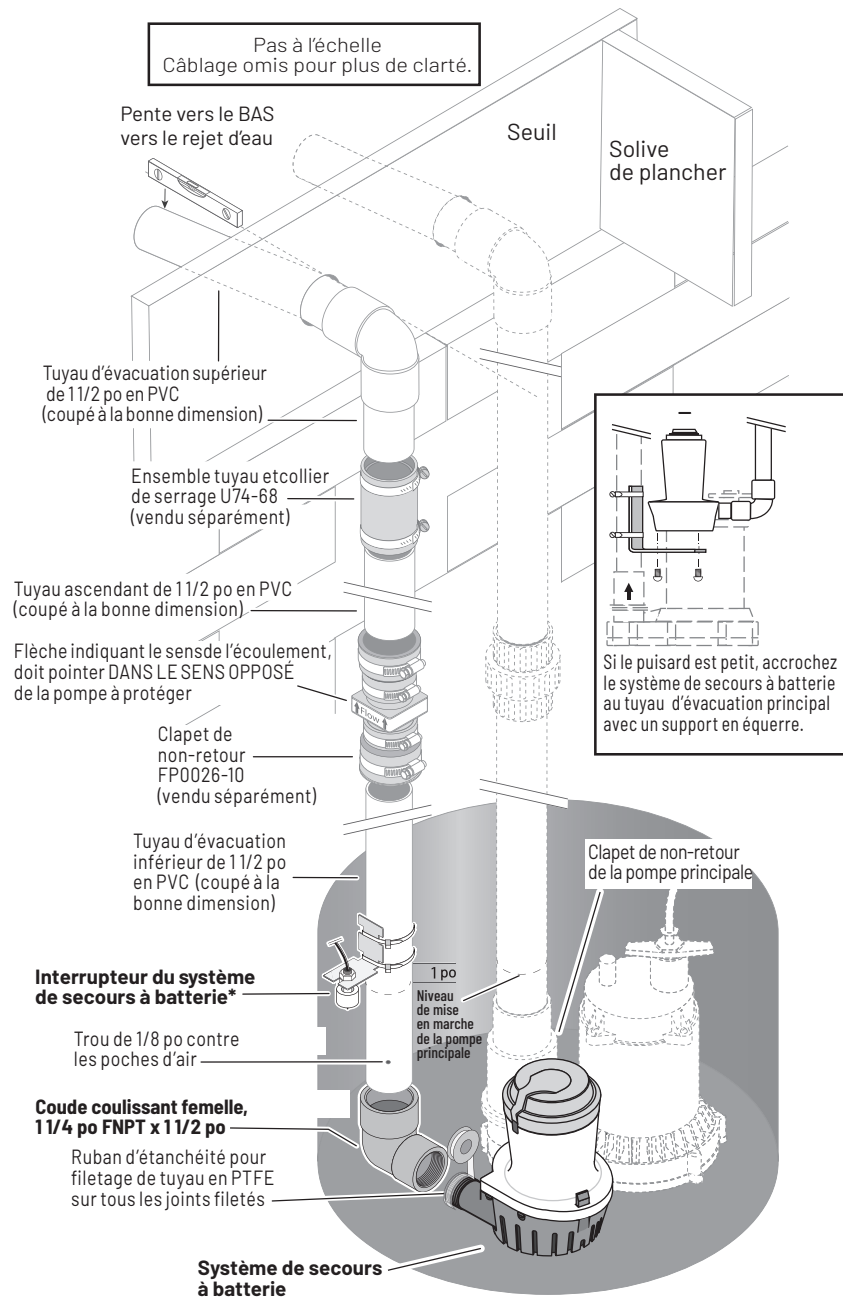
Figure 2 : Évacuation séparée – Installation type
