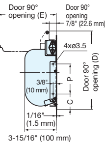
AZ-GD230-HL AZ-GD230-BL
