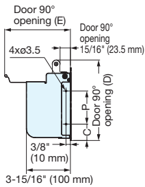
AZ-GD180-HL
